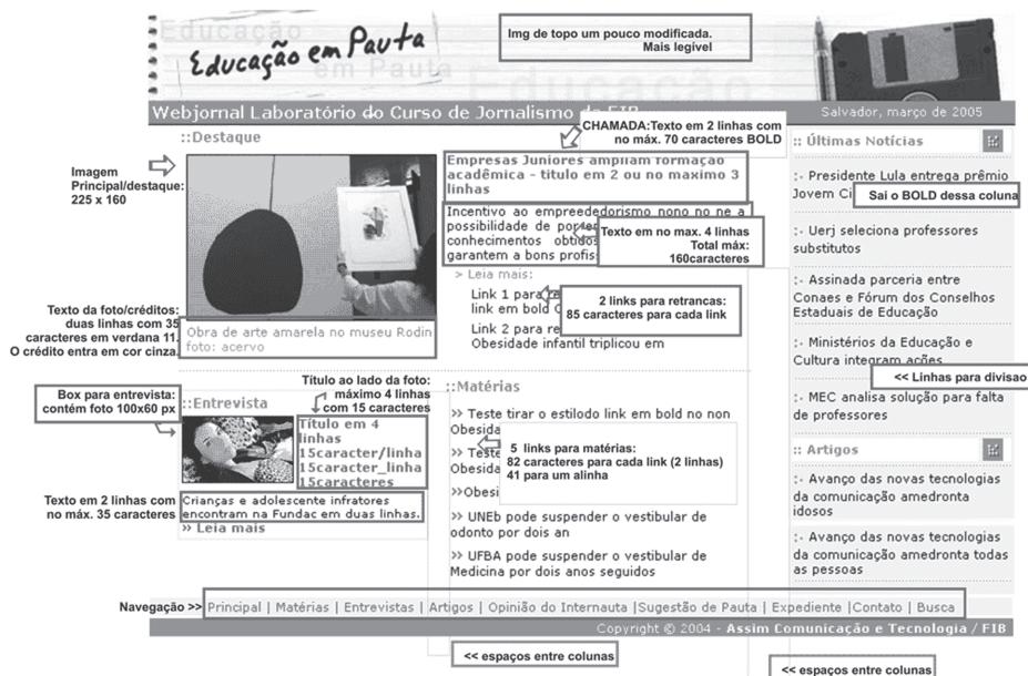
Figura 3 – Projeto reestruturado em 2004.2
